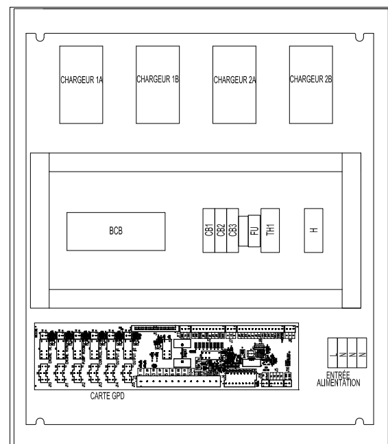
AGENCEMENT INTERNE
