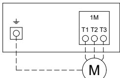
Terminales de motor
